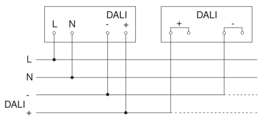
Schema elettrico collegamento in rete di DALI-2 APC & DALI-2 IPD
